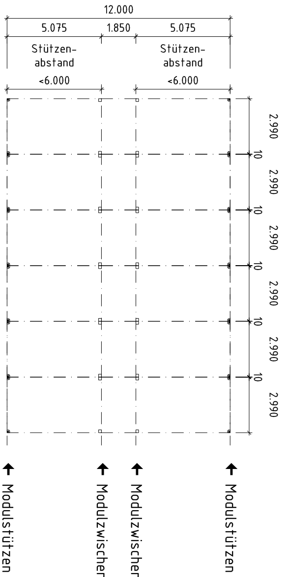
Statisches Systembeispiel Gebäudebreite 12m
